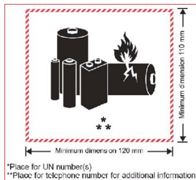
图 3：锂电池操作标签
